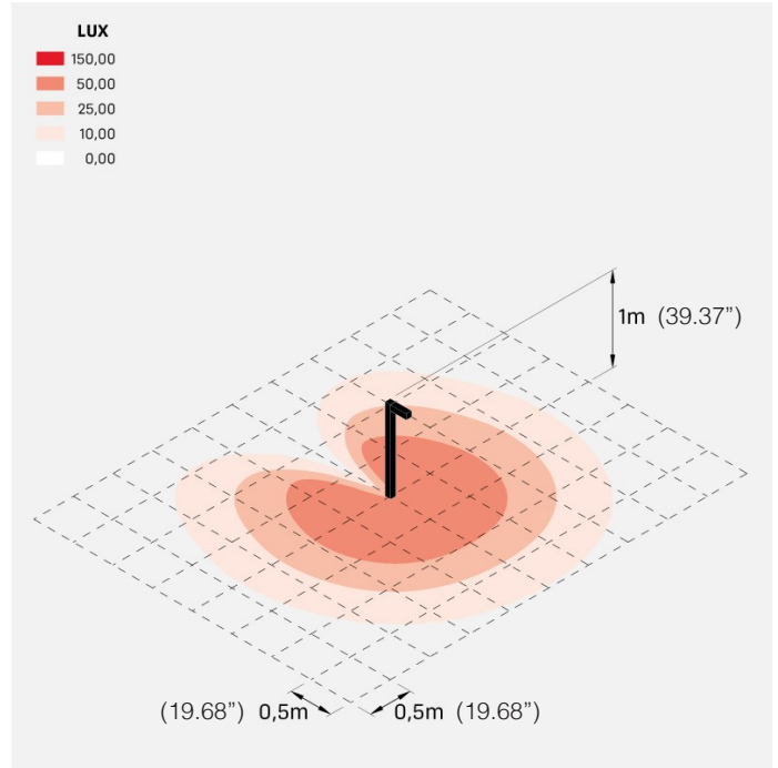
silvio 200_bollard_w
