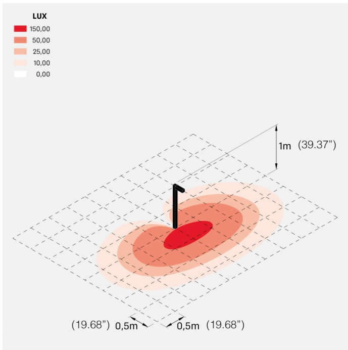
silvio 200_bollard_a
