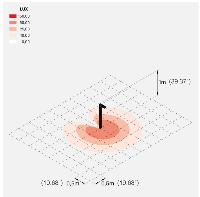
silvio 200_bollard_d
