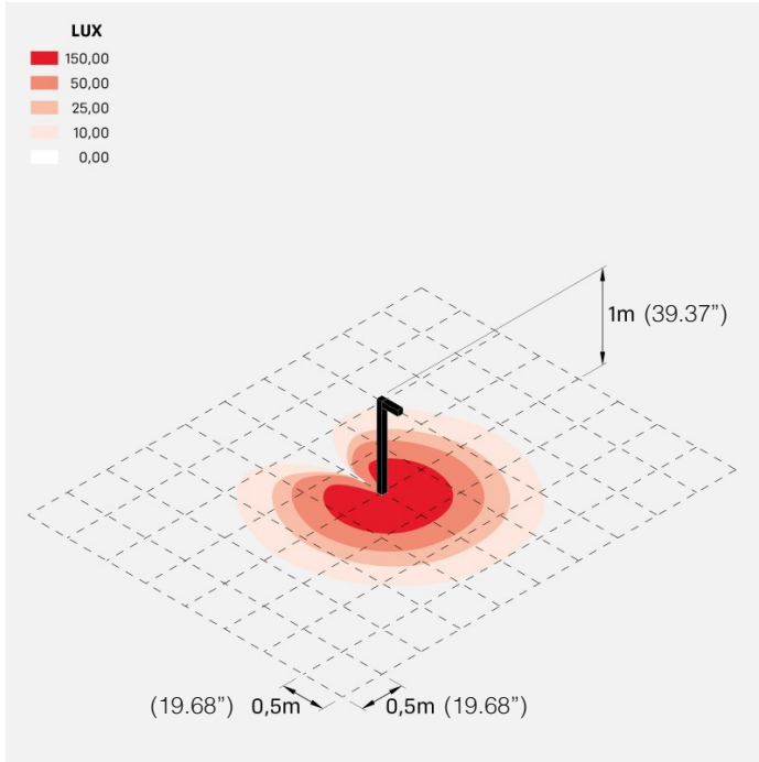
silvio 200_bollard_s
